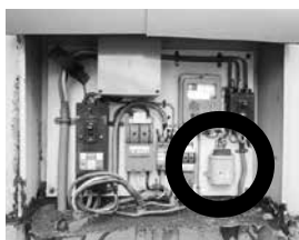
変圧器
