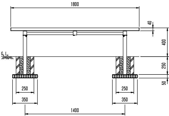
正面図 (S=1/20)
