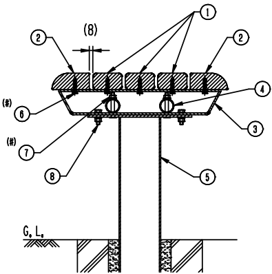
組付断面図 (A-A矢視図) (S=1/10)
