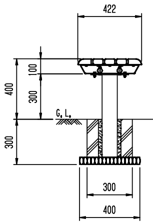
側面図 (S=1/20)
