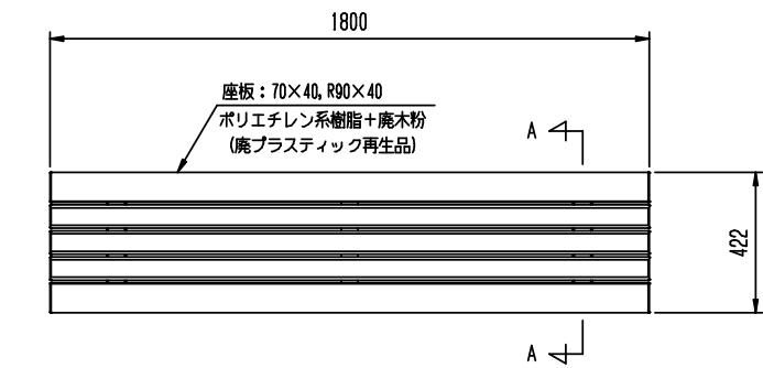
平面図 (S=1/20)
