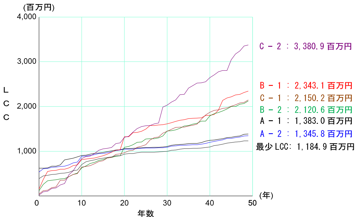
図 5-11 シナリオ別 LCC 算定結果
