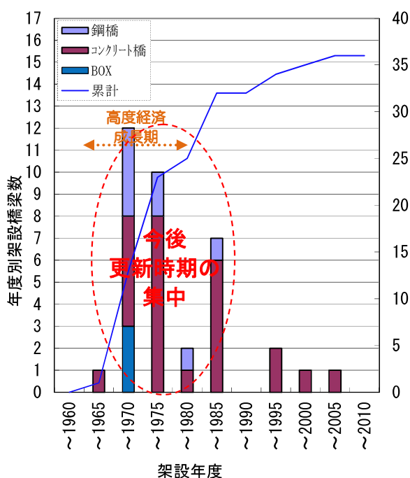
図 1-1 今別町橋梁の状況
